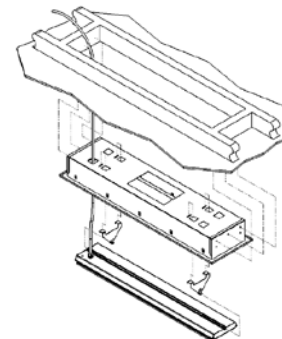
Montage omhulsel voor inbouw Boîtier encastrable
